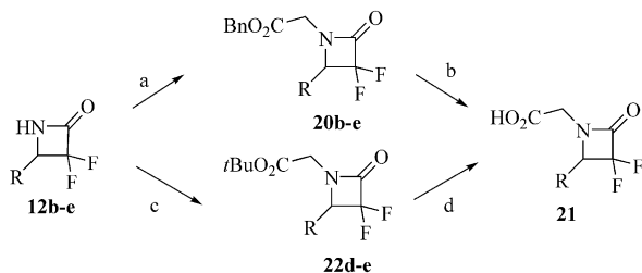
Scheme 11. (a) \text{BrCH}_2\text{CO}_2\text{Bn} , TMG, TBAI, MeCN, room temp.; (b) \text{H}_2 , Pd/C, EtOH, room temp.; (c) \text{BrCH}_2\text{CO}_2t\text{Bu} , TMG, TBAI, MeCN, room temp.; (d) TFA, \text{CH}_2\text{Cl}_2 , 0^\circ\text{C} .
